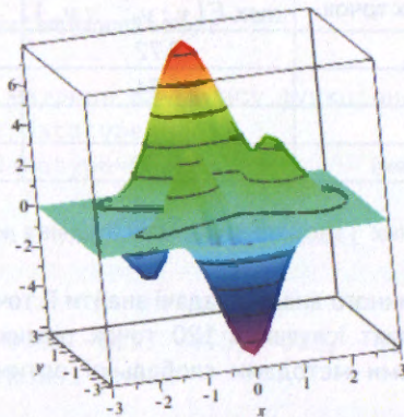
Рисунок 1 - Графік функції (14)
