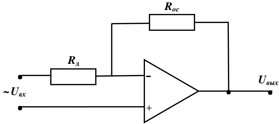
Рис. 2. Схема определения связи сопротивления датчика влажности и напряжения на выходе операционного усилителя ( U_{vyx} – напряжение, снимаемое с выхода операционного усилителя; U_{vx} – напряжение, подведенное к датчику; R_d – сопротивление датчика влажности; R_{oc} – сопротивление резистора обратной связи)
