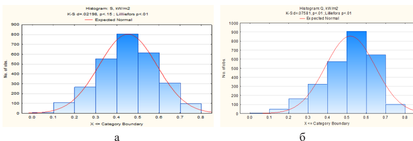
Рис. 2. Емпіричні закони розподілу прямої (а) та сумарної (б) сонячної радіації в м. Херсоні за період 1981–2010 рр.
