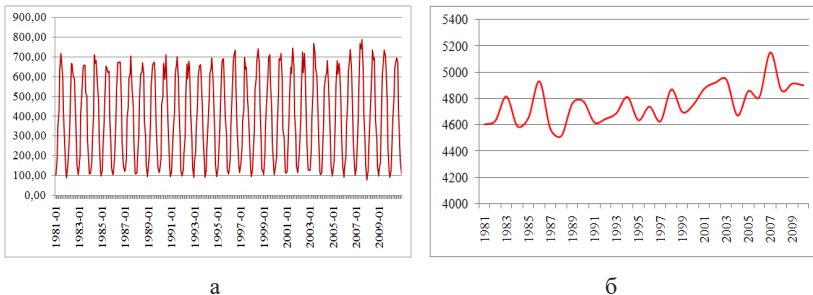
Рис. 1. Багаторічний хід сумарної сонячної радіації у м. Херсоні: а) місяць (МДж/м 2 ); б) рік (МДж/м 2 )
