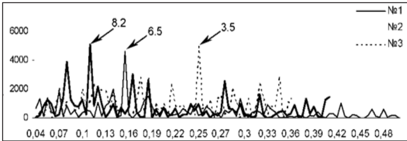
Рис. 1. Щільність дендрохронологічних рядів сосни звичайної: сосняк чорнично-моховий – 1; сосняк сфайгновий – 2; сосняк чорничний – 3
