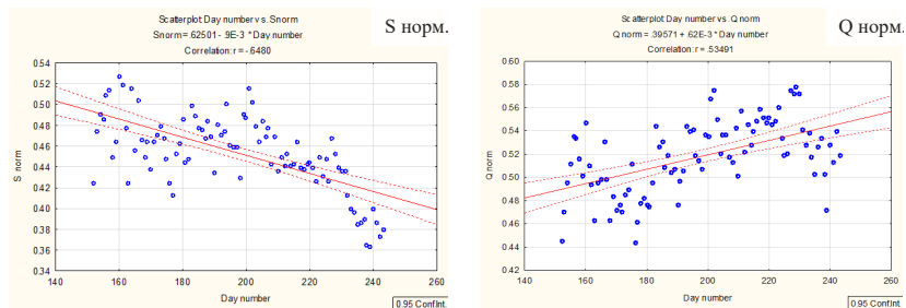
Рис. 4. Динаміка нормованих значень прямої та сумарної сонячної радіації в м. Херсоні за період 1981–2010 рр.
