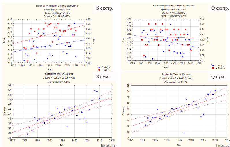
Рис. 3. Динаміка екстремальних значень і сум прямої та сумарної сонячної радіації в м. Херсоні за період 1981–2010 рр.
