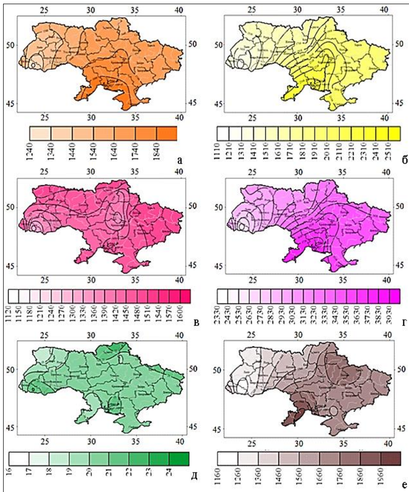
Рис. 1. Тривалість сонячного сйва (год) (а), пряма (МДж/м 2 ) (б), розсіяна (МДж/м 2 ) (в) і сумарна (МДж/м 2 ) сонячна радіація (г), альbedo (%) (д) і радіаційний баланс підстильної поверхні (МДж/м 2 ) (е) у 1991–2020 рр. за теплий період року
