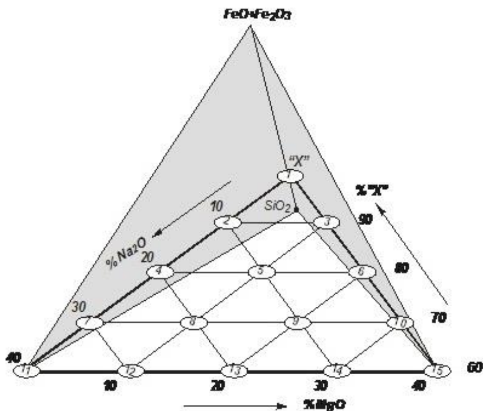
Рисунок 1. Схема вибору складів стекол у системі (Fe_2O_3-FeO)-SiO_2-MgO-Na_2O
