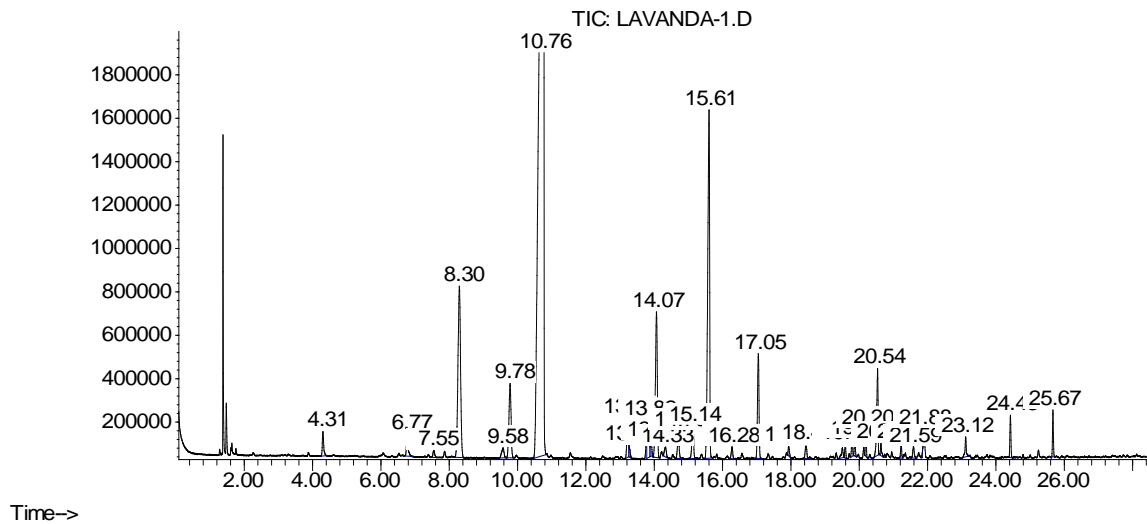
Рис. 4. Хроматограма ефірної олії із суцвіть Lavandula hybrida Rev. сорт Іній, 2018 р.
