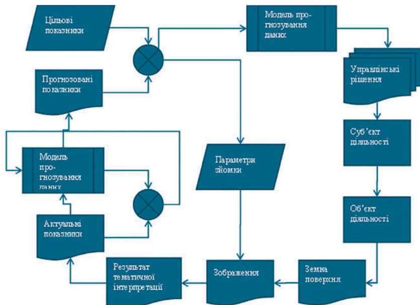
Рис. 2. Узагальнена схема системи обробки геопросторової інформації
