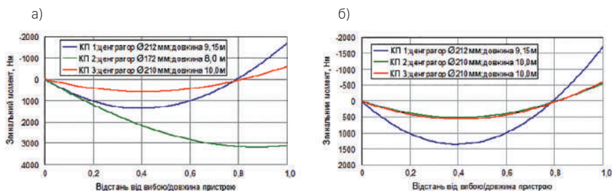
Рис. 5. Розподіл згинальних моментів в односекційних керноприймальних пристроях КП1, КП 2, КП 3 (пояснення в тексті):
