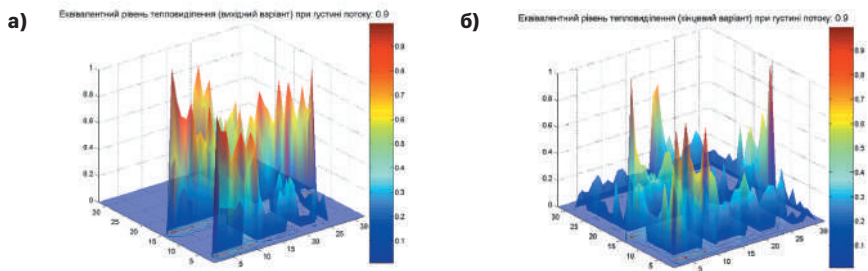
Рис. 1. Еквівалентний рівень тепловиділення, спричиненого роботою двигунів автомобілів на перехресті: а) до вдосконалення схеми дорожнього руху; б) після введення об'їзної дороги
