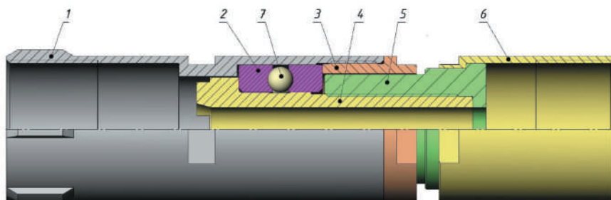
Рис. 3. Підшипниковий підвіс з центрувальними елементами:
