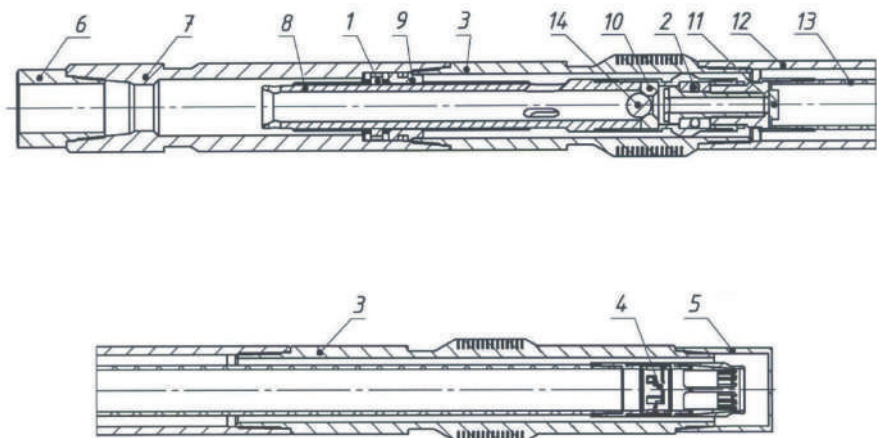
Рис. 1. Система подовженого керноприймального пристрою:
