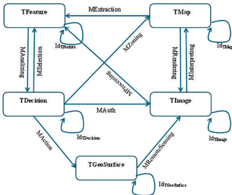
Рис. 3. Основні об'єкти та морфізми системи обробки геопросторової інформації
