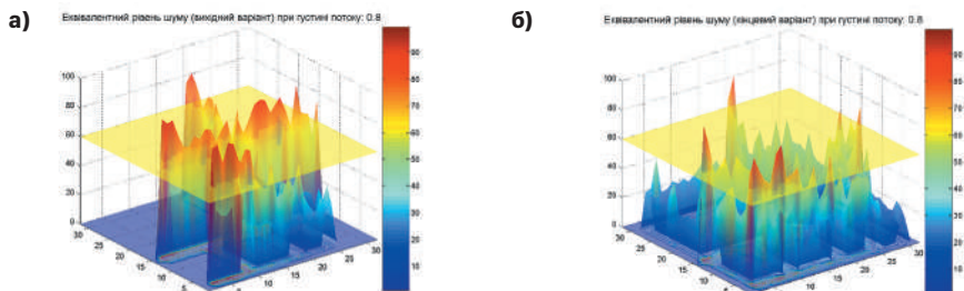
Рис. 2. Еквівалентний рівень шуму, створюваного автомобілями на перехресті: а) до вдосконалення схеми дорожнього руху; б) після введення об'їзної дороги
