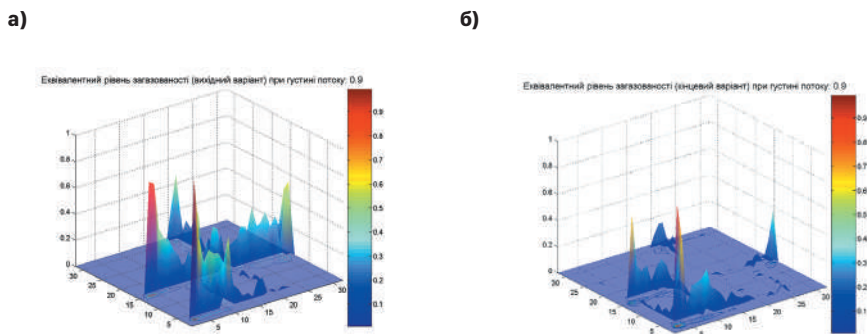
Рис. 3. Еквівалентний рівень загазованості, викликаній автомобілями на перехресті: а) до вдосконалення схеми дорожнього руху; б) після введення об'їзної дороги
