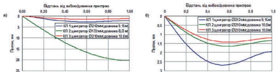
Рис. 4. Розподіл прогинів односекційних керноприймальних пристроїв КП 1, КП 2, КП 3 (пояснення в тексті):
